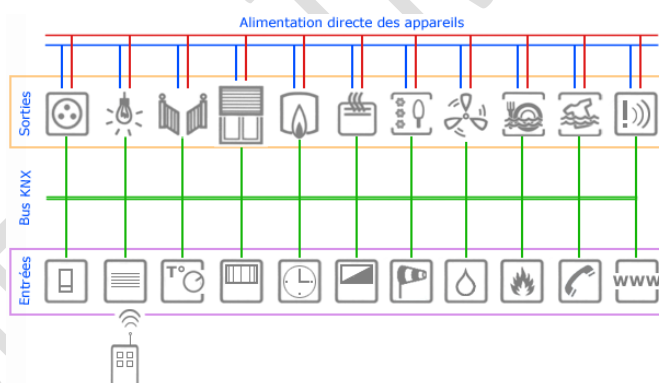
Principe de câblage d'un réseau KNX
